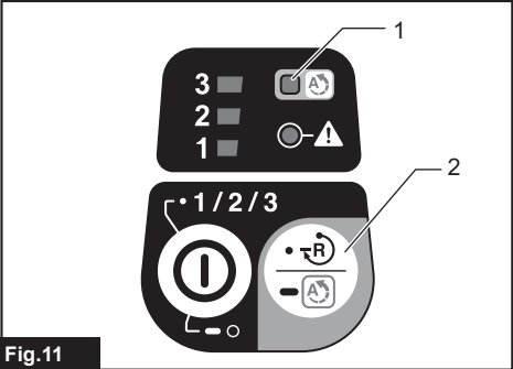
Fig.11 ► 1. Indicador de ADT 2. Botón de inversión
